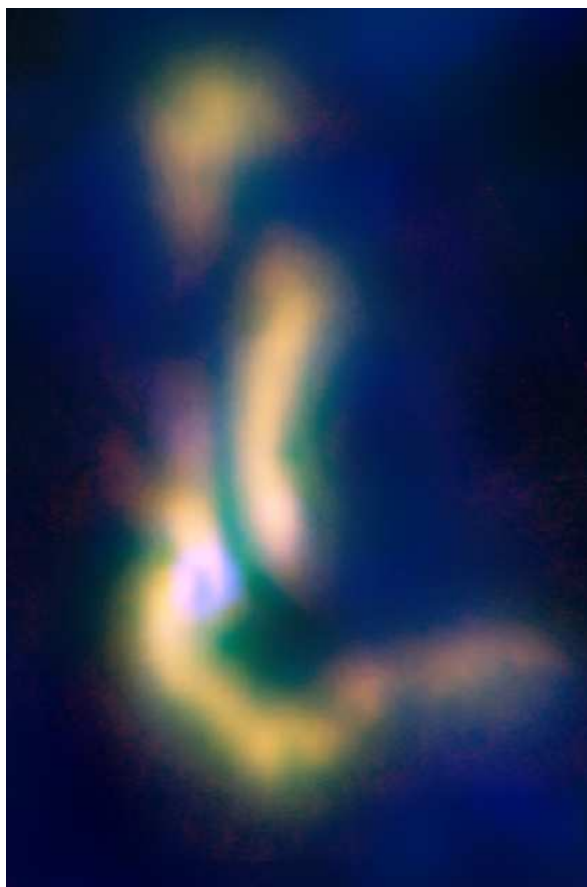
La nube di gas B5, ripresa nella fase di formazione stellare: diventerà un sistema multiplo di stelle. Crediti: NRAO/AUI/NSF
