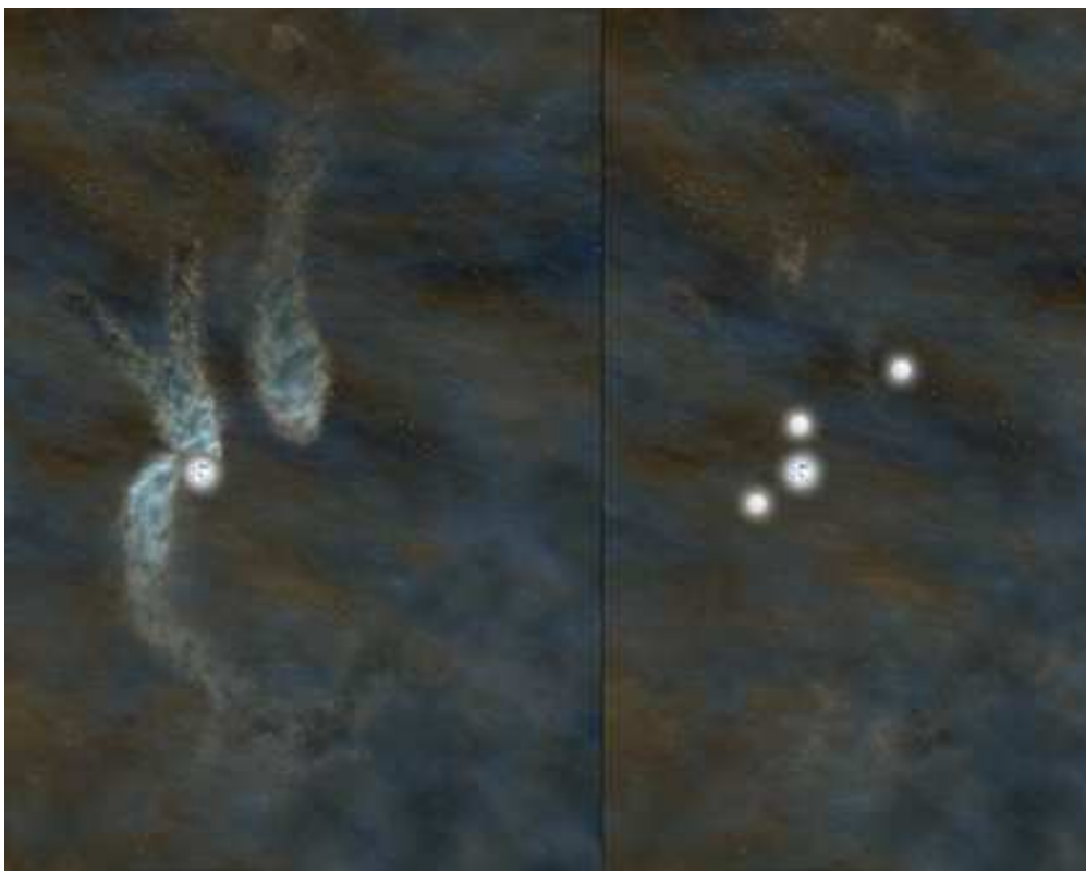
Rappresentazione artistica di come B5 come appare oggi, a sinistra, e di come apparirà fra circa 40.000 anni quando si sarà formato il sistema multiplo di stelle, a destra. Crediti: Bill Saxton, NRAO/AUI/NSF
