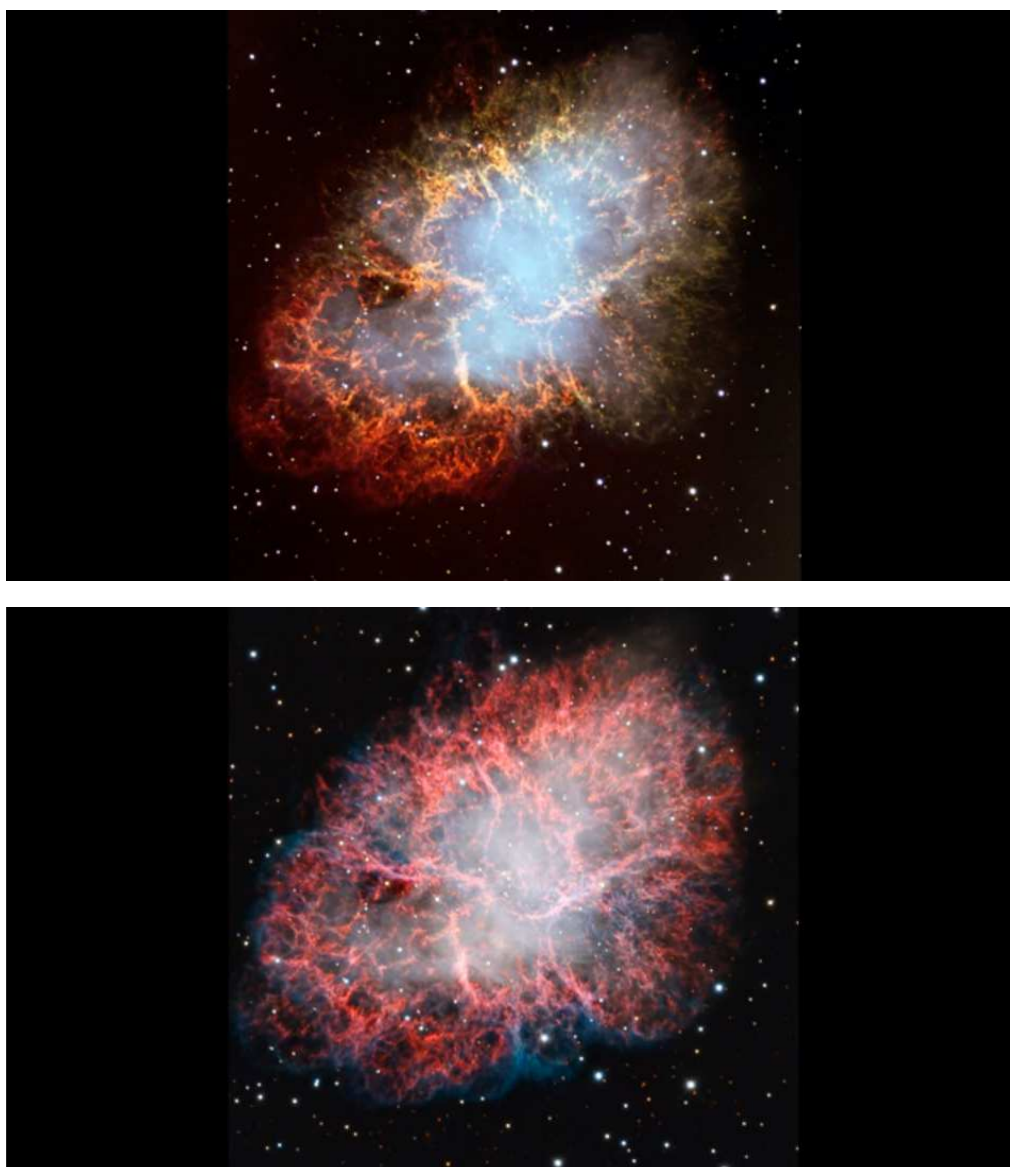
La Crab Nebula (M1) nel 1999 e nel 2012.
