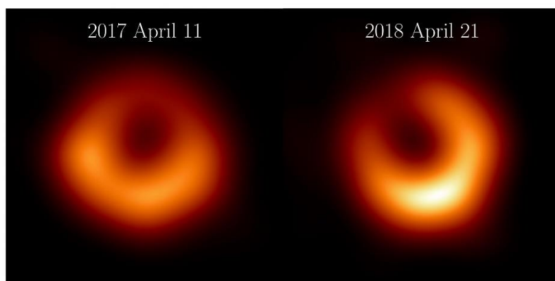
La nuova immagine del buco nero al centro della galassia M87 (sulla destra) confrontata con quella ottenuta dalle prime osservazioni della stessa sorgente (sulla sinistra). Crediti: Collaborazione Eht
