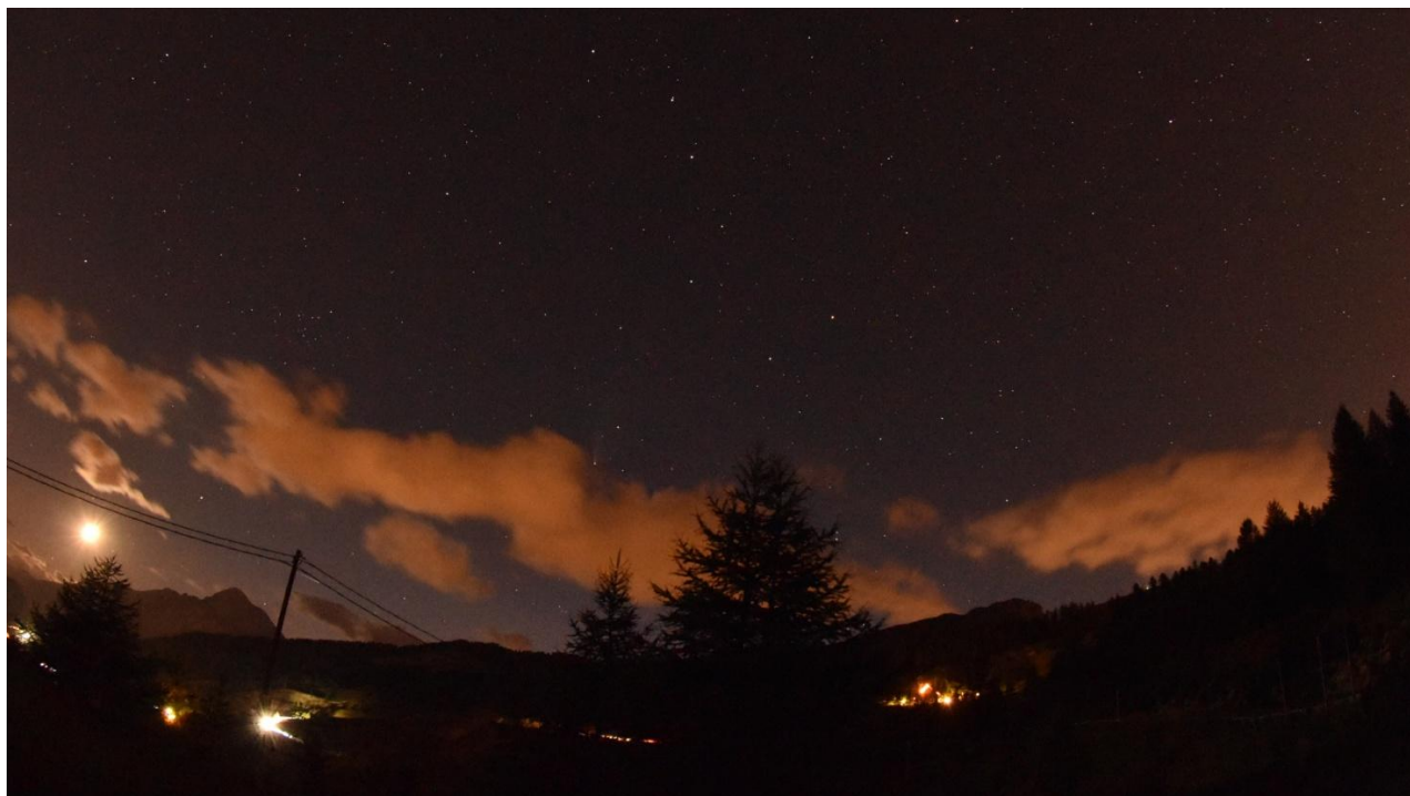
Cometa NEOWISE (C/2020 F3) il 24 luglio 2020 alle ore 21:56 CEST da Grangesises (TO), 1859 m slm, con Nikon D5500, 10 mm, f/5.6, 13 s, 6100 ISO. A sinistra la Luna al tramonto. (Andrea Ainardi)
