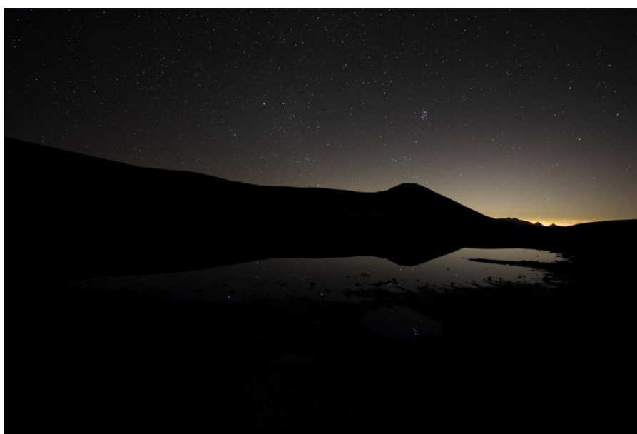
A sinistra, le Pleiadi si specchiano nel piccolo lago di fronte al Rifugio; a destra, la Via Lattea si staglia sopra al Rifugio (7-8 settembre 2018). Fotocamera Canon EOS 60D, fisheye 14 mm, 30 s, 1600 ISO (a sinistra) e 3200 ISO (a destra), posa fissa su treppiede. (Immagini di Alessio Gagnor)
