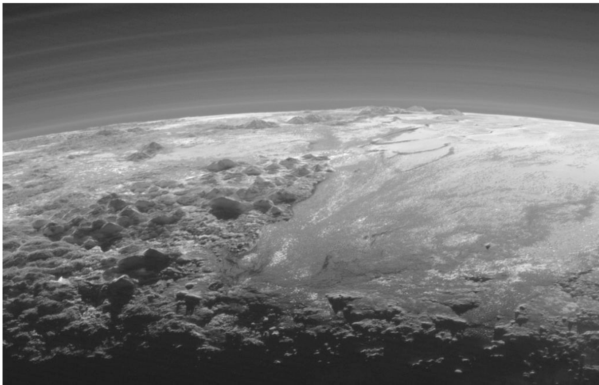
Particolare dell'immagine precedente: la scena ha 380 chilometri di larghezza. Crediti: NASA / JHUAPL / SwRI
