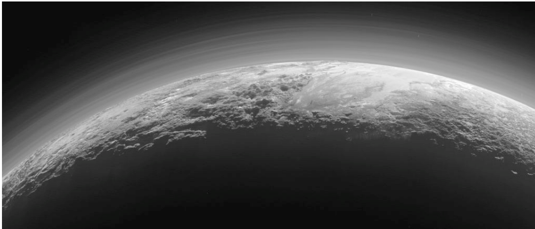
Plutone ripreso da New Horizons il 14 luglio scorso da una distanza di 18.000 chilometri: la scena ha 1.250 chilometri di larghezza. Crediti: NASA / JHUAPL / SwRI
